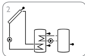
Sistema de energía solar con intercambio de calor (página 11)
