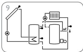
Sistema de energía solar con aumento de la temperatura de retorno del circuito de calefacción (página 40)
