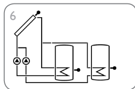
Sistema de energía solar con 2 acumuladores y lógica de bomba (página 28)
