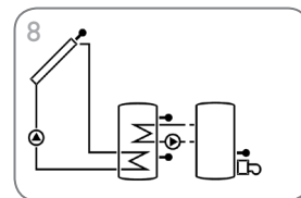
Sistema de energía solar con calentamiento auxiliar por caldera de biomasa (página 34)
