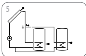
Sistema de energía solar con 2 acumuladores y lógica de válvula (página 25)
